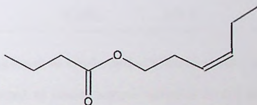
(Z)-3-hexenyl butanoate
