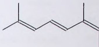
Allo-ocimene
