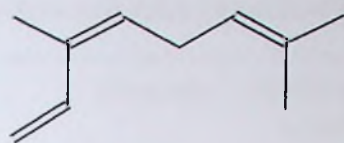
(Z)-β-ocimene
